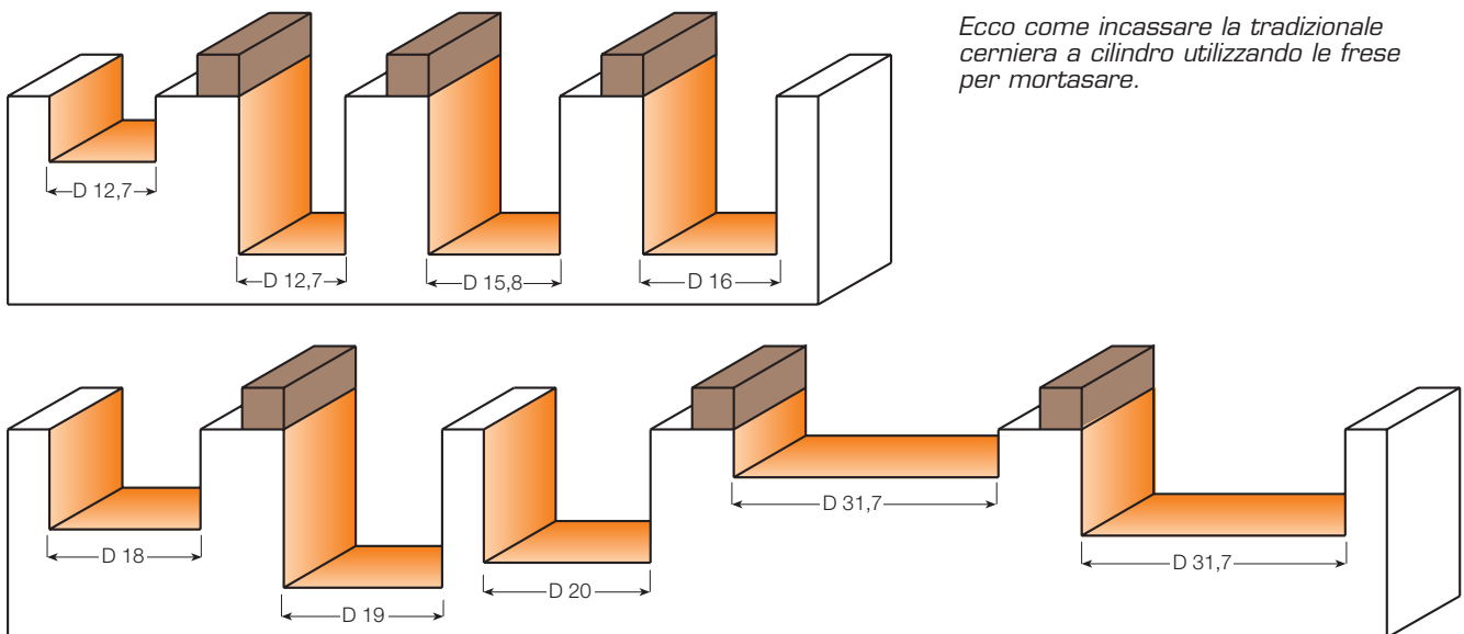
Profili in scala 1:1
