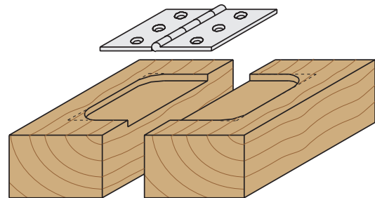
Ecco come incassare la tradizionale cerniera a cilindro utilizzando le frese per mortasare.
