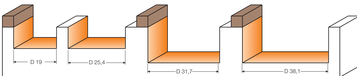
Profili in scala 1:1
